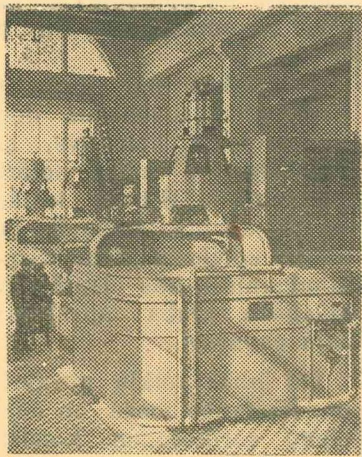
Attēlā: jaunās HES mašīnu zāle.
