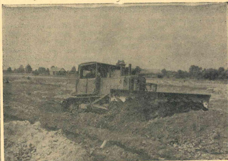
Attēlā: drenu grāvju aizbērsšana ar slīpo traktorlāpstu.
