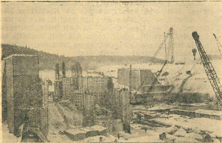
Ufimskas HES būvlaukumā patreiz norit armatūras celtniecības darbi un betonēšana. Attēlā: Ufimskas HES slūžu apakšējā daļa.
